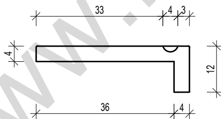
ISTRA II sa zubom 40cm; l=60cm
